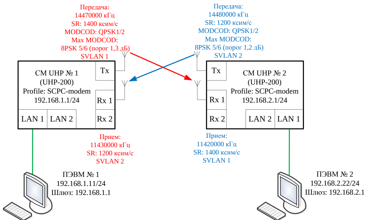
Рисунок 2. Сеть топологии «точка-точка», построенная на CM UHP-200 в составе ЗССС Ку-диапазона
